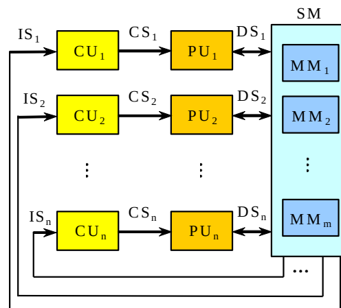
(d) MIMD 计算机
